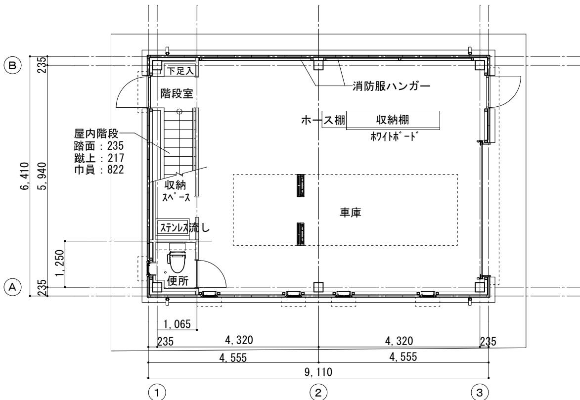
1階平面図 1/100
