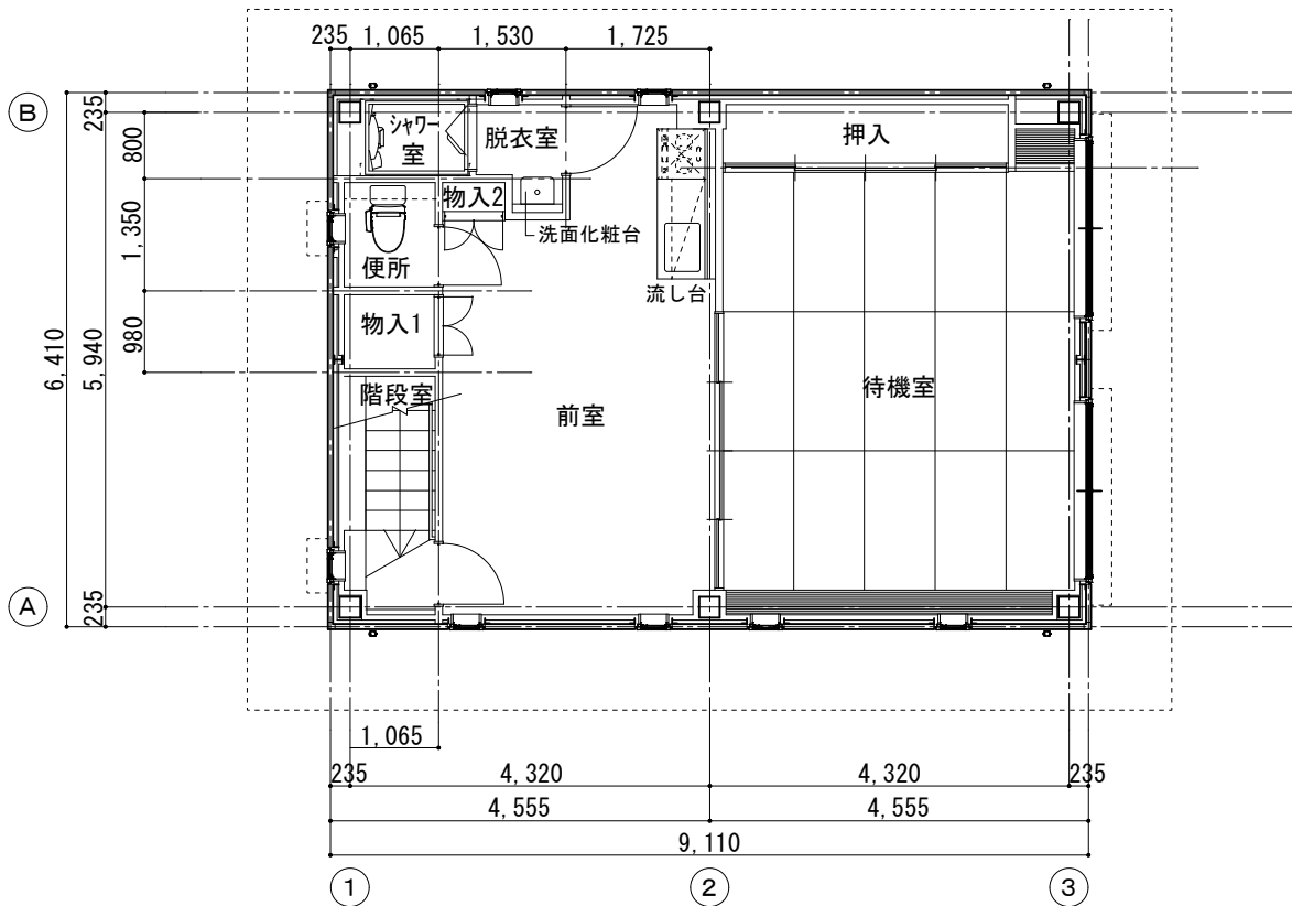
2階平面図 1/100
