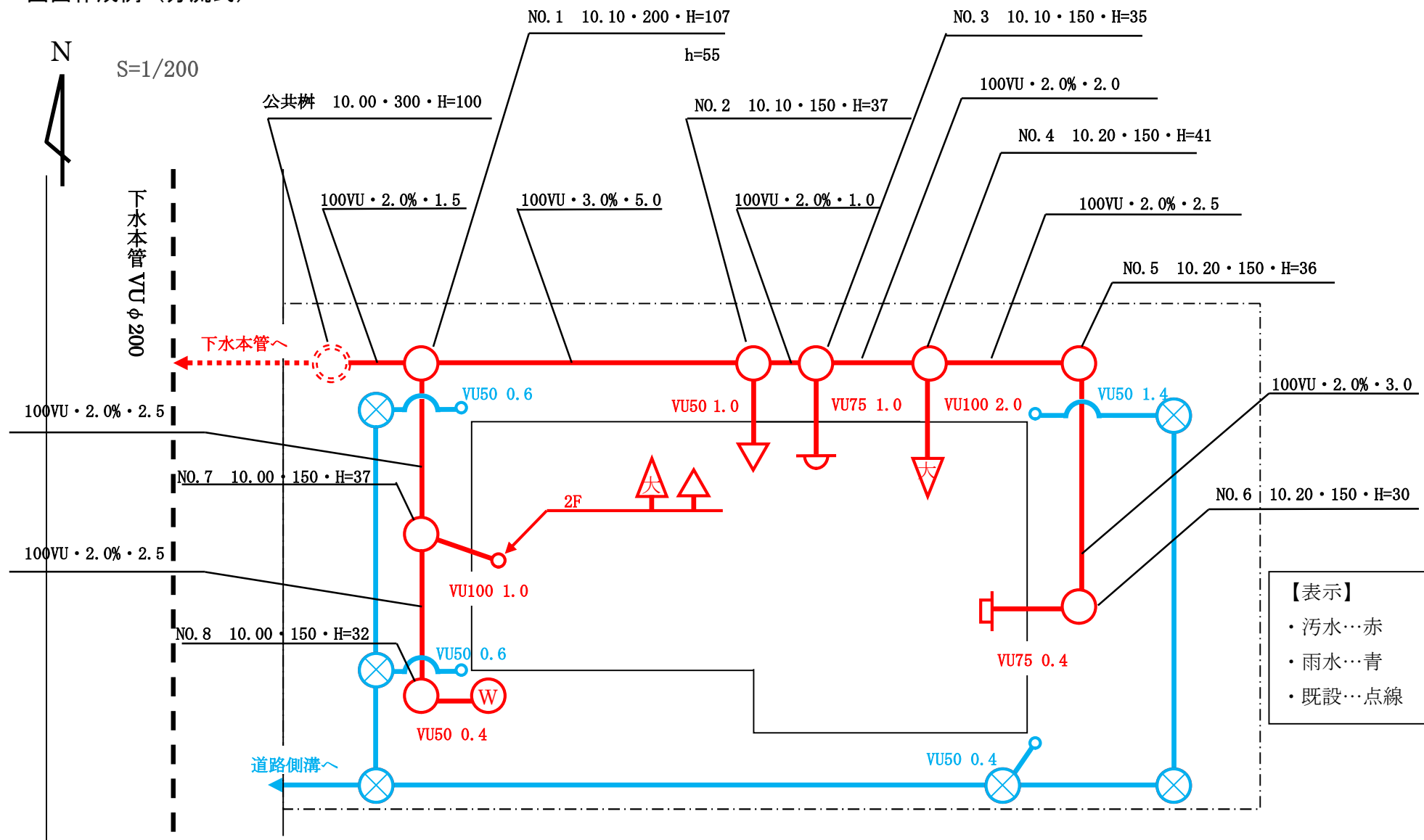
図面作成例（分流式）
