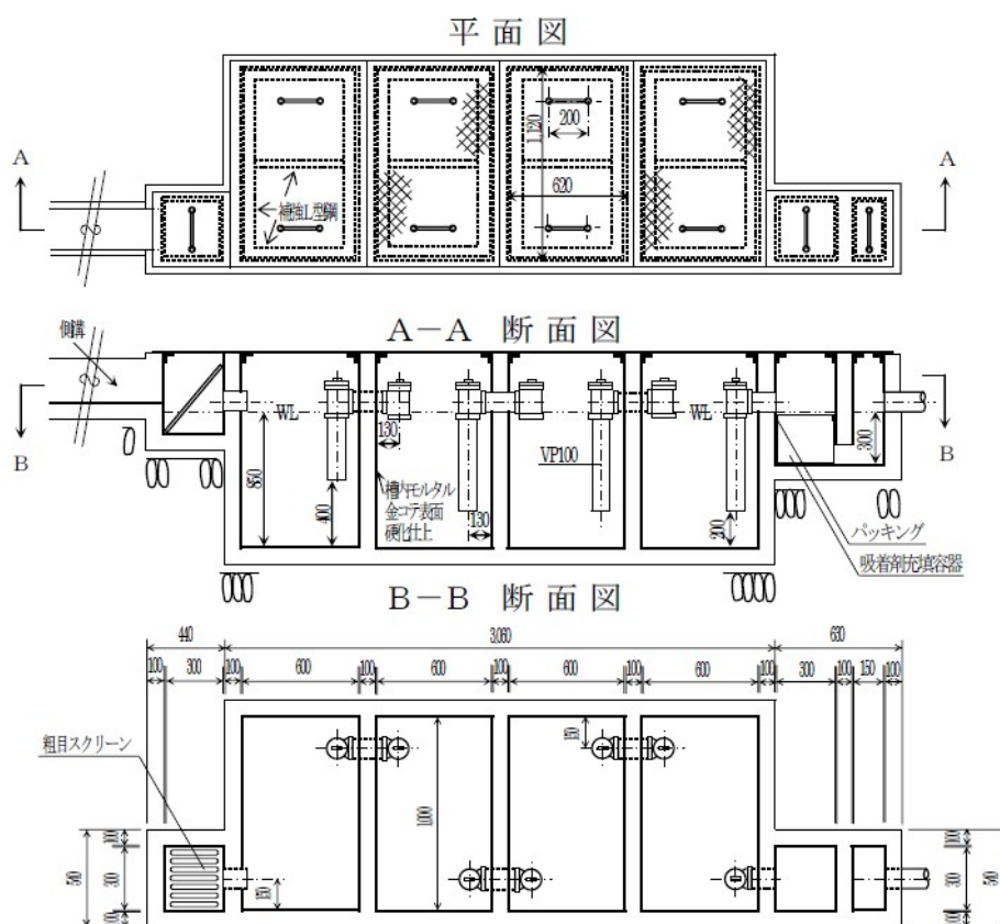
油水分離槽（基本構造）
