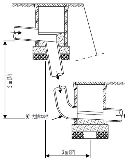
底部有孔ますの一例
